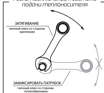
Рис. 3. Подключение к системе подачи теплоносителя
