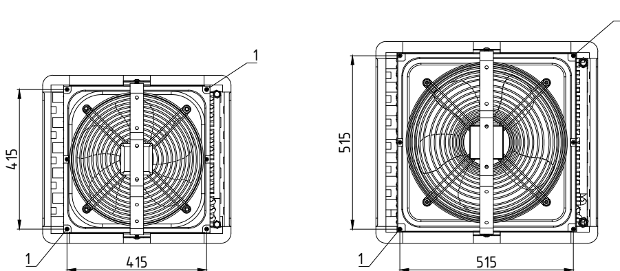
Рис. 3. Расстояния между крепежными держателями
